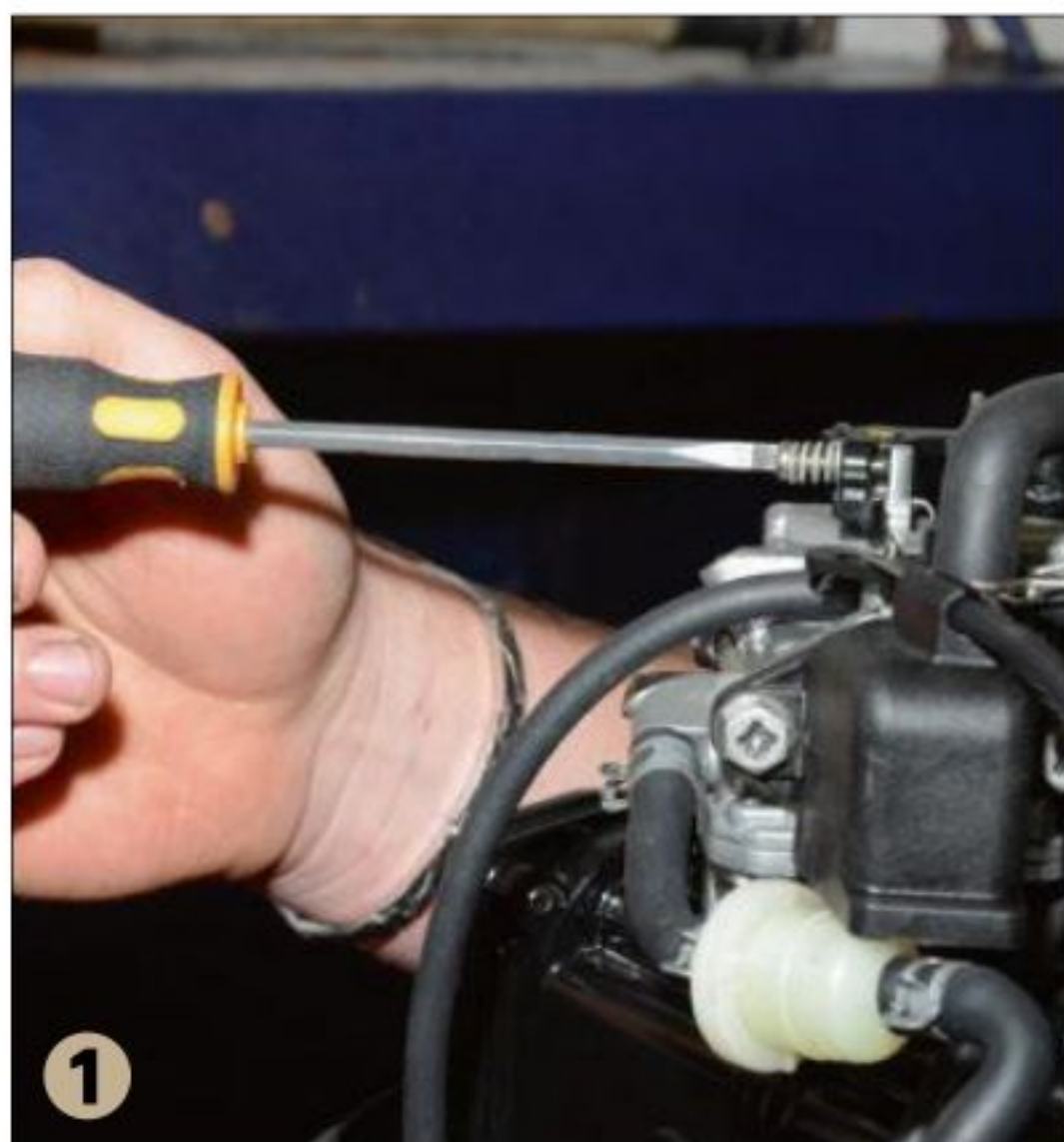
1 ▲ Après avoir fait chauffer le moteur pendant une dizaine de minutes, on règle d'abord le ralenti avec la vis dédiée (celle avec un ressort), jusqu'à obtenir un régime d'environ 1 500 tr/mn.
